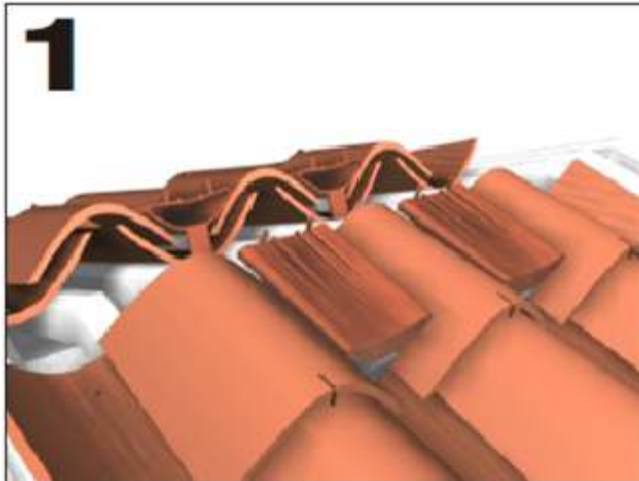
1 Posa bocchette su malta
