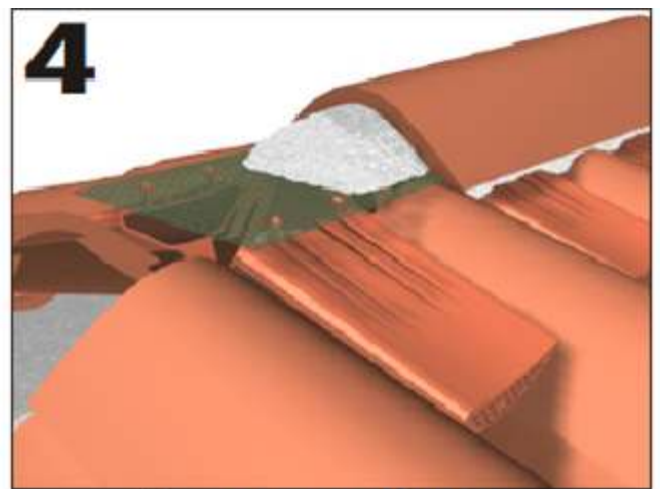
4 Posa coppo di colmo
